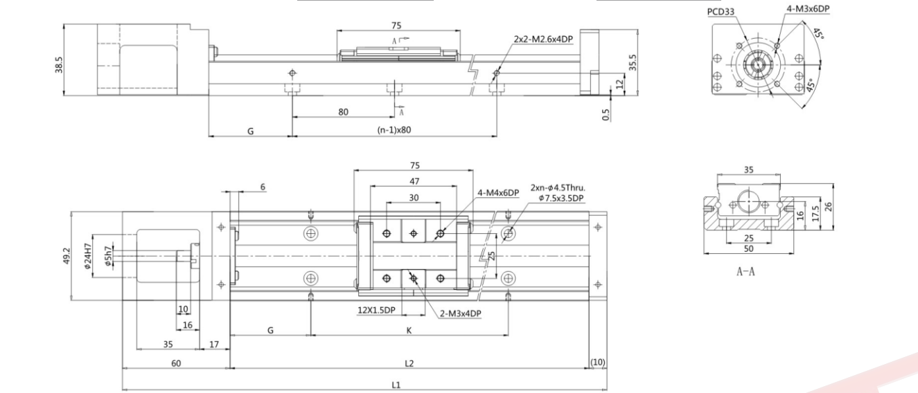
PKK50直线模组-尺寸图 PKK50-TECHNICAL PARAMETER
